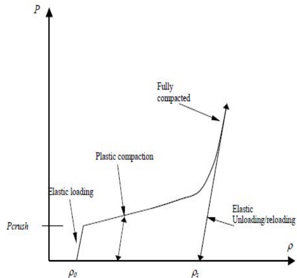
شکل ۳. نمودار رفتار چگالی-فشار بتن [۱۱]
