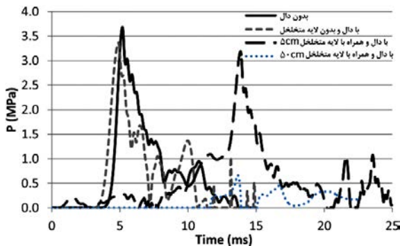
شکل ۱۴. تغییرات فشار در فاصله ۳ متری از انفجار در شرایط مختلف دال
