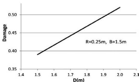
شکل ۲۵. توزیع خسارت بر حسب تغییرات فاصله چاه‌ها از دیوار
