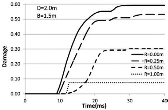
شکل ۲۰. پیشرفت خسارت در بحرانی‌ترین نقطه روی دیواره سازه در شرایطی که فاصله چاه‌ها از یکدیگر ۱/۵ متر و از دیواره سازه ۲ متر می‌باشد.
