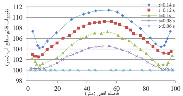
شکل ۱۱. منحنی تغییرات سطح آب با زمان (روش SPH)
