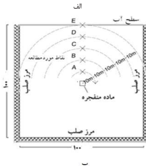
شکل ۵. الف- هندسه مدل مورد مطالعه ب- نحوه قرارگیری ذرات در روش SPH
