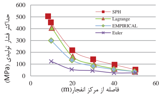
شکل ۱۰. مقایسه حداکثر فشار تولیدی روش SPH با روش تجربی و دیدگاه‌های لاگرانژی و اولری
