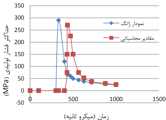
شکل ۴. مقایسه نتایج مدل‌سازی عددی با روش بدون شبکه و نتایج ژانگ
