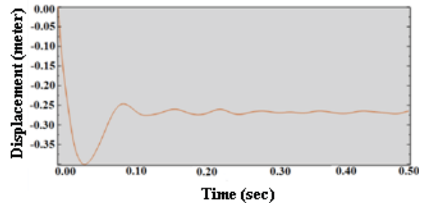
شکل ۱۰. تغییر شکل وسط شاه تیر دوم پل ۱۵ متری تحت بار انفجار ۱۰۰۰ پوند TNT (۴۵۴ کیلوگرم TNT)
