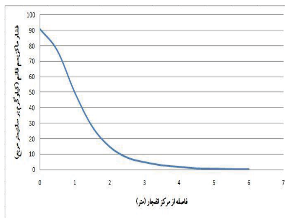
شکل ۳. فشار پیک قائم برای خرج انفجار ۲۵۰ پوند TNT
