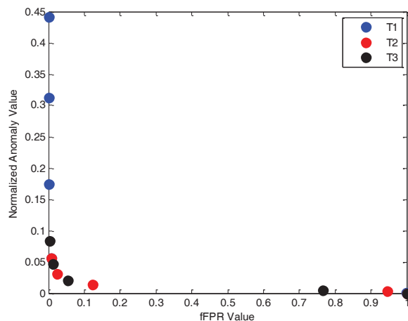
شکل ۱۶. عدد ناهنجاری (محور عمودی) و پارامتر fFPR (محور افقی) مربوط به سطوح مختلف استتاری اهداف واقعی چندپیکسلی در تصویر منطقه شهری در تگزاس
