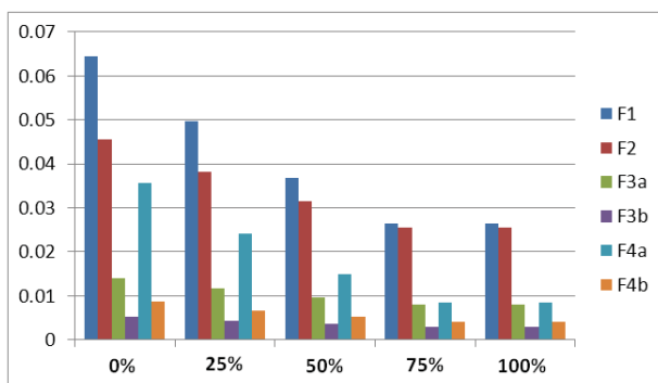
شکل ۵. عدد ناهنجاری (محور عمودی)، در مقابل کسر (درصد) استتار شده از پیکسل هدف (محور افقی)
