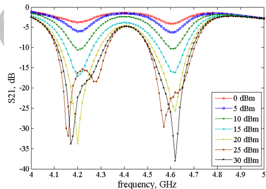
شکل ۱۳. S_{21} محدودکننده مبتنی بر فرکانس اصلاح‌شده.
