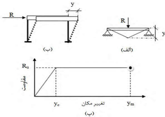
شکل ۱. سازه یک درجه آزادی الاستوپلاستیک [۵]
