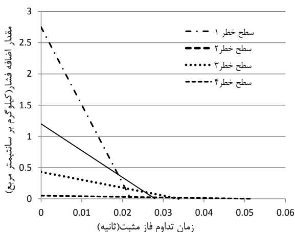
شکل ۶. نمودار فشار- زمان برای سطوح خطر چهارگانه
