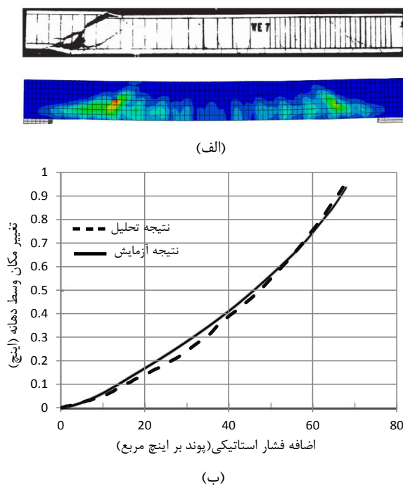
شکل ۹. مقایسه نتایج آزمایشگاهی با مدل عددی تیر WE7 تحت بار استاتیکی- الف) الگوی ترک، ب) تغییر مکان وسط دهانه تیر
