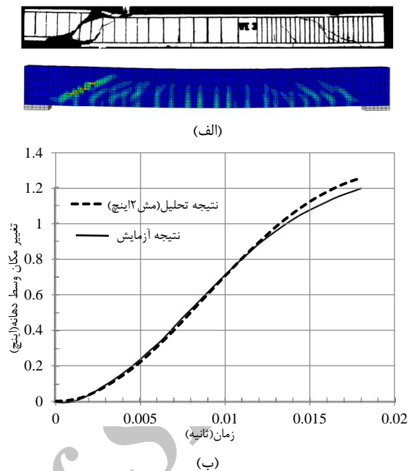
شکل ۷. مقایسه نتایج آزمایشگاهی با مدل عددی تیر WE3 تحت بار انفجار با المان چهار وجهی (C3D8R)، الف) الگوی ترک، ب) تغییر مکان وسط دهانه
