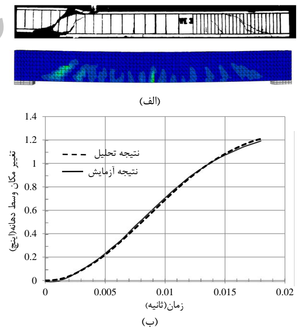
شکل ۸. مقایسه نتایج آزمایشگاهی با مدل عددی تیر WE3 تحت بار انفجار با المان سه رأسی (C3D4)، الف) الگوی ترک، ب) تغییر مکان وسط دهانه
