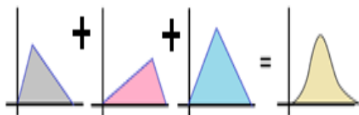
شکل ۹. تجمیع توابع توزیع مثلثی
