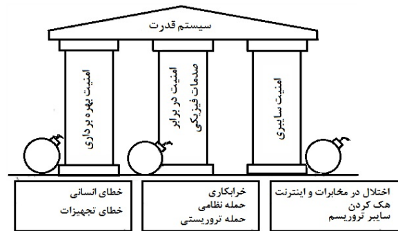
شکل ۱. ابعاد مسئله امنیت سامانه قدرت [۱۰]
