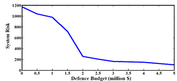
شکل ۱۶. منحنی کاهش ریسک سامانه به ازای افزایش بودجه پدافندی
