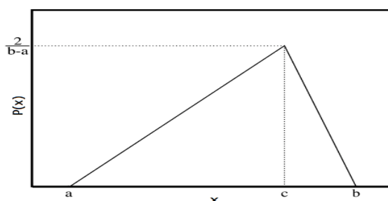
شکل ۷. تابع چگالی احتمال تابع توزیع مثلثی
