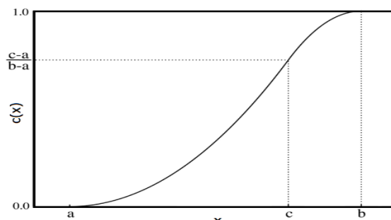
شکل ۸. تابع توزیع تجمعی تابع توزیع مثلثی
