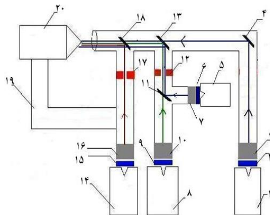
شکل ۱۱. طراحی سخت‌افزار آزمونگر پیشنهادی
