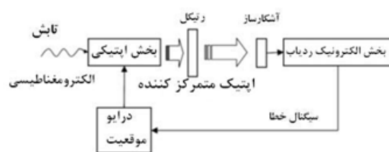
شکل ۳. دیاگرام بلوکی یک جستجوگر رتیکلی [۱۰]
