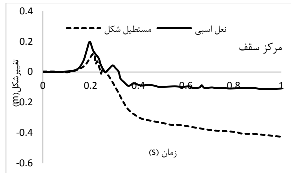
شکل ۸. تغییر شکل در مرکز دیوار و مرکز سقف
