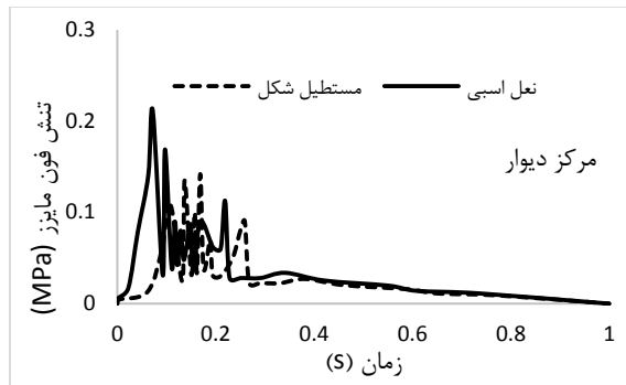
شکل ۷. تنش فون مایزر در المان‌های تاج و مرکز دیوار دو تونل در عمق ۱۰ متری
