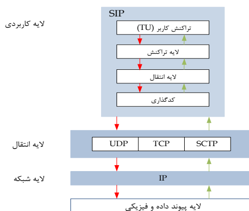
شکل ۱. ساختار لایه‌ای و حالت‌مند SIP در لایه کاربردی [۴]
