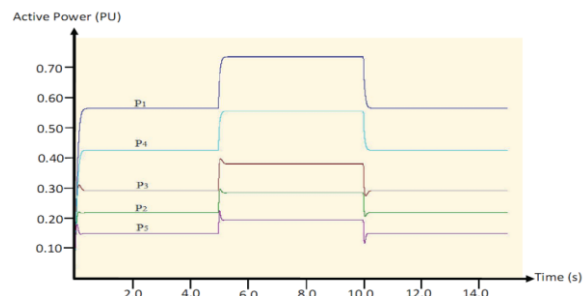
شکل ۹. توان تولیدی توسط واحدهای VSC در ریزشبه جزیره‌ای گسترش یافته
