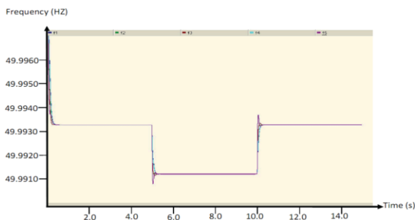
شکل ۱۱. فرکانس خروجی واحدهای VSC در ریزشبه جزیره‌ای گسترش یافته
