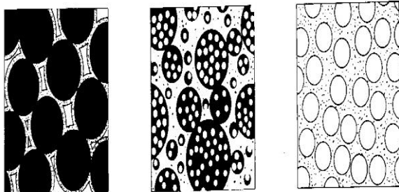
شکل ۱. سه نوع پایه‌ای انواع مختلف بتن سبک. بتن بدون ریزدانه بتن سبک دانه بتن هوادار
