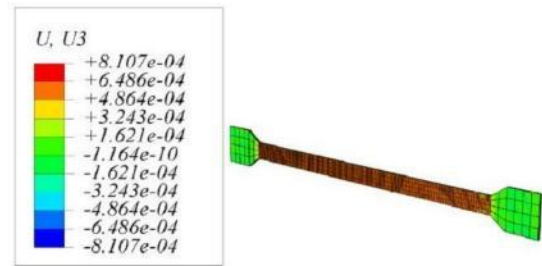
شکل ۱۷. تغییر مکان مدل سه بعدی هسته مقید شده به وسیله فنر تحت بارگذاری انفجار بر حسب متر
