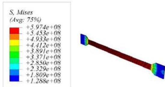
شکل ۱۳. تغییرات تنش بر اساس معیار فون میسز در هسته تحت بار انفجار 1 Blast بر حسب پاسکال
