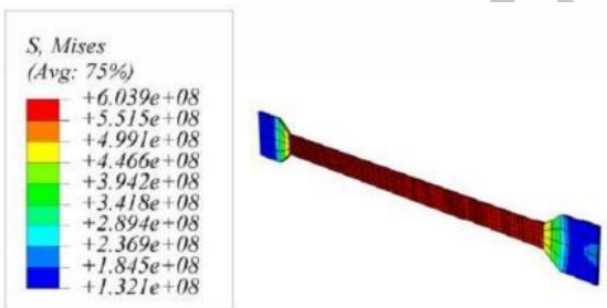
شکل ۱۵. تغییرات تنش بر اساس معیار فون میسز در هسته تحت بار انفجار 3 Blast بر حسب پاسکال
