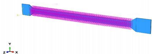
شکل ۳. مدل سه‌بعدی هسته و فنر در پژوهش حاضر
