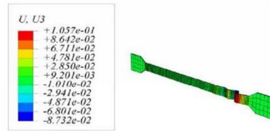
شکل ۱۸. تغییر مکان مدل سه بعدی هسته بدون قید جانبی تحت بارگذاری انفجار بر حسب متر
