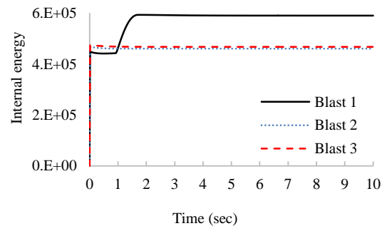
شکل ۲۱. نمودار تاریخچه زمانی انرژی داخلی مهاربند کمانش‌ناپذیر تحت بار انفجار
