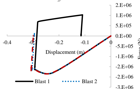
شکل ۱۶. منحنی بار- جابه جایی مدل سه بعدی هسته مقید شده تحت بارگذاری انفجار
