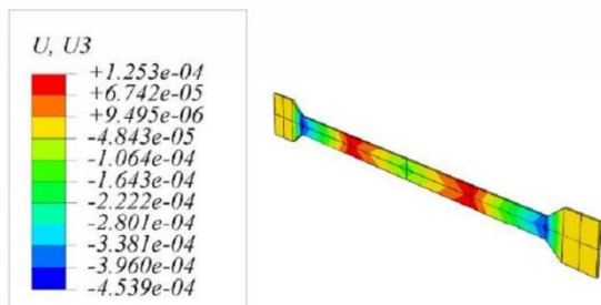
شکل ۶. تغییر مکان مدل سه‌بعدی هسته مقید شده توسط فنر تحت بارگذاری حوزه نزدیک SAC بر حسب متر
