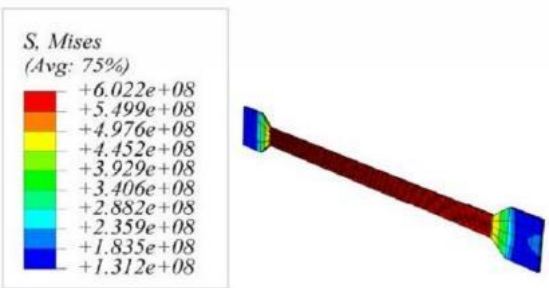
شکل ۱۴. تغییرات تنش بر اساس معیار فون میسز در هسته تحت بار انفجار 2 Blast بر حسب پاسکال
