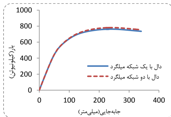
شکل ۱۳. نمودار بار- جابه‌جایی قاب با یک و دو شبکه میلگرد تحت حذف ستون گوشه
