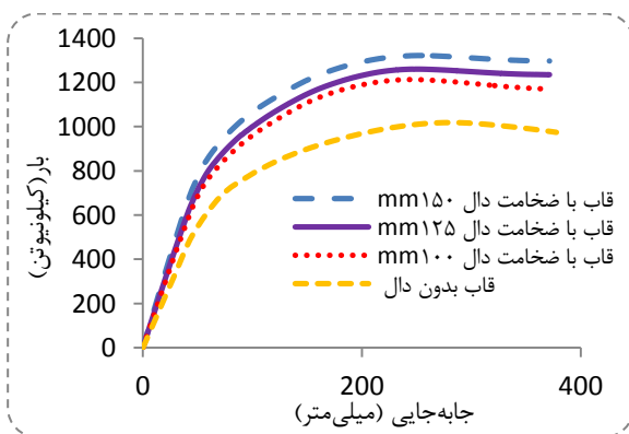
شکل ۱۴. نمودار بار - جابه‌جایی حاصل از حذف ستون کناری با ضخامت‌های مختلف دال
