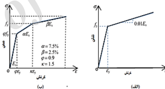
شکل ۴. نمودار تنش-کرنش مصالح مورد استفاده: (الف) فولاد و (ب) میلگرد [۱۶]
