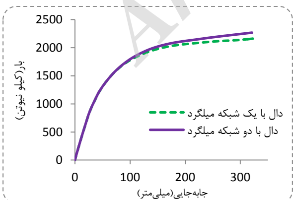
شکل ۱۹. نمودار بار- جابه‌جایی قاب با یک و دو شبکه میلگرد تحت حذف ستون میانی
