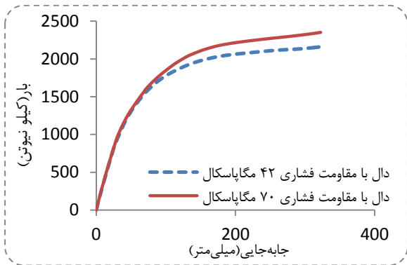
شکل ۱۸. نمودار بار- جابه‌جایی قاب با مقاومت فشاری مختلف تحت حذف ستون میانی
