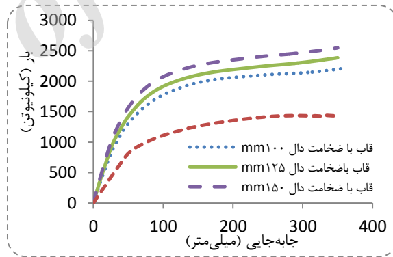
شکل ۱۷. نمودار بار - جابه‌جایی حاصل از حذف ستون میانی با ضخامت‌های مختلف دال
