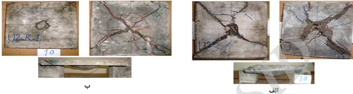
شکل ۹. الگوی گسیختگی نهایی؛ (الف) پانل U-S و (ب) پانل U-R؛ (راست) وجه پشتی و (چپ) وجه جلویی
