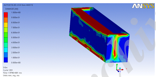
شکل ۱۰. میزان خرابی مدل شماره ۳
