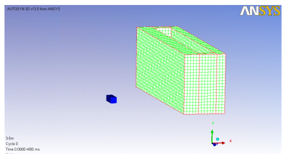
شکل ۷. مش‌بندی مدل مورد مطالعه
