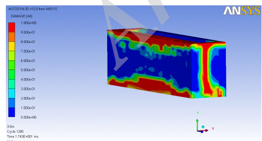
شکل ۱۱. میزان خرابی مدل شماره ۴
