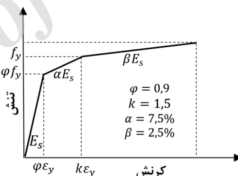
شکل ۴. نمودار تنش-کرنش میل‌گرد مورد استفاده [۱۴]
