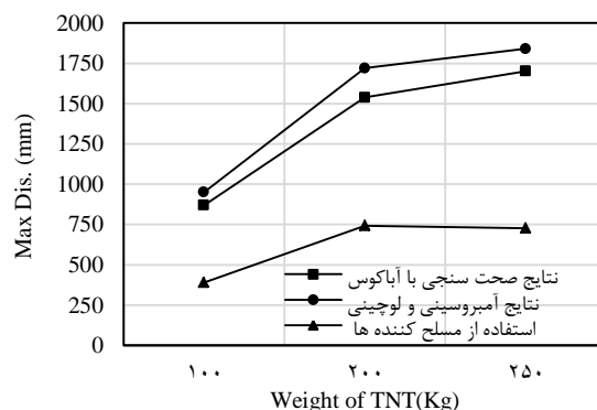
شکل ۹. نمودار بین شدت انفجار و عمق چاله انفجاری در خاک مسلح
