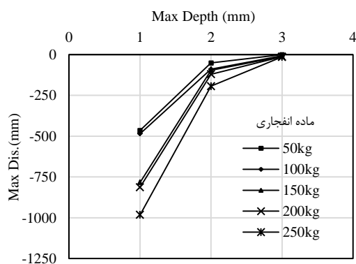
شکل ۱۲. نمودار جابه‌جایی تاج لوله ناشی از انفجار
