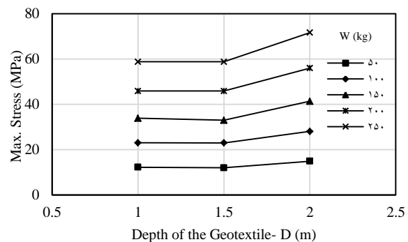
شکل ۱۶. نمودار تنش حداکثر در لوله نسبت به عمق مسلح‌کننده مدفون در خاک
