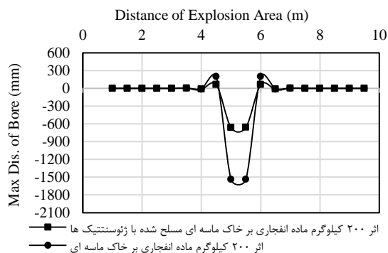
شکل ۱۰. تفاوت تغییر شکل چاله انفجاری خاک با استفاده و بدون استفاده از مسلح‌کننده‌ها تحت اثر بار انفجاری ۲۰۰ کیلوگرم TNT
