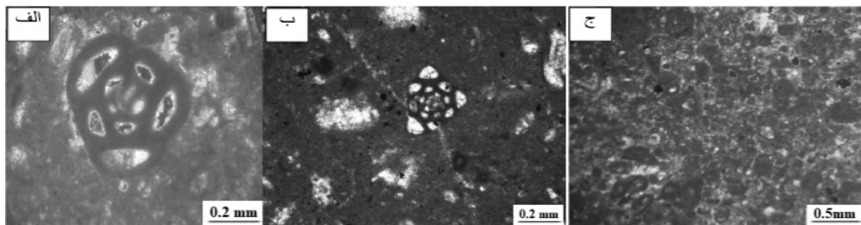
شکل ۷ تصاویر میکروسکوپی از تأثیر فرآیند میکربیتی شدن در کربنات‌های سازند ایلام: الف- تشکیل پوشش میکربیتی در اطراف میلیولید در رخساره وکستون؛ ب- تشکیل پوشش میکربیتی در اطراف فرامینفر بنتیک در رخساره وکستونی؛ ج- میکربیتی شدن پلوئیدها در رخساره پکستون پلوئیدی.
