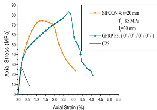
شکل ۱۹: نمودار تنش- کرنش هسته بتنی به مقاومت ۲۵ مگاپاسکال، محصور شده توسط طرح های محصورسازی S4 و F5
