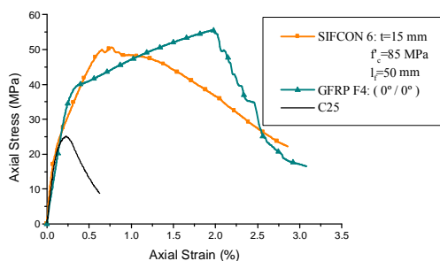
شکل ۱۷: نمودار تنش-کرنش هسته بتنی به مقاومت ۲۵ مگاپاسکال، محصور شده توسط طرح های محصورسازی S6 و F4
