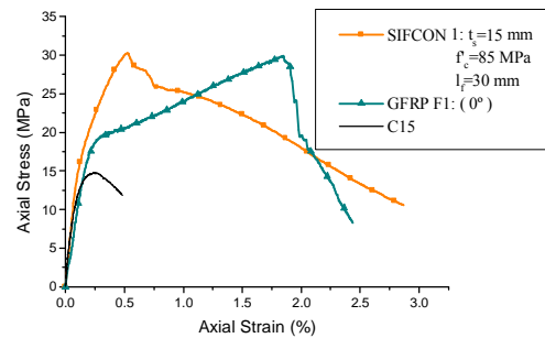
شکل ۱۵: نمودار تنش-کرنش هسته های بتنی به مقاومت ۱۵ مگاپاسکال، محصور شده توسط طرح های محصورسازی S1 و F1
