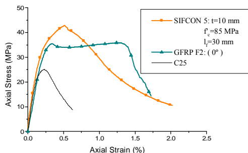
شکل ۲۰: نمودار تنش- کرنش هسته بتنی به مقاومت ۲۵ مگاپاسکال، محصور شده توسط طرح های محصورسازی S5 و F2
