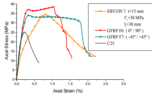
شکل ۱۸: نمودار تنش- کرنش هسته بتنی به مقاومت ۲۵ مگاپاسکال، محصور شده توسط طرح های محصورسازی S7 و F7, F6
