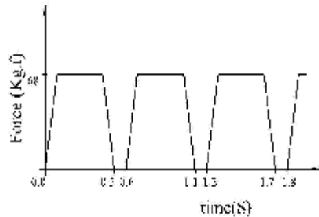
شکل ۶: بارگذاری قدم زدن روی دال.
