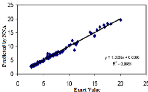
شکل ۳: همبستگی نتایج واقعی و نتایج پیشگویی شده توسط شبکه برای بسامد دوم.
