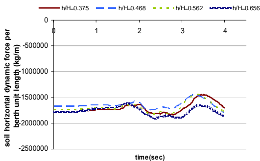
شکل ۵: نیروی کل جانبی دینامیکی خاک پشت دیوار در چهار مدل با نسبت h/H مختلف.
