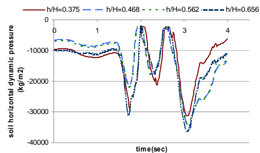
شکل ۴: فشار جانبی دینامیکی خاک پشت بلوک بالایی در مدل‌های با نسبت h/H مختلف.
