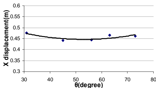
شکل ۷: جا به جایی افقی نهایی بلوک بالایی مدل‌های بر حسب زاویه گوژ.
