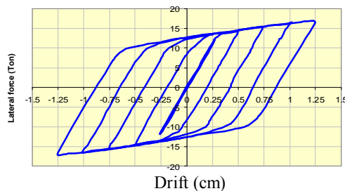
شکل ۵: منحنی هیستریزیس قاب KBF 2.
