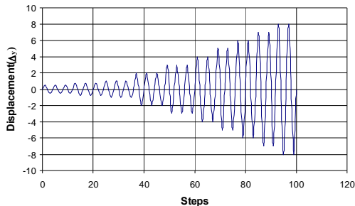
شکل ۳: بارگذاری چرخه ای AISC-LRFD 1997.
