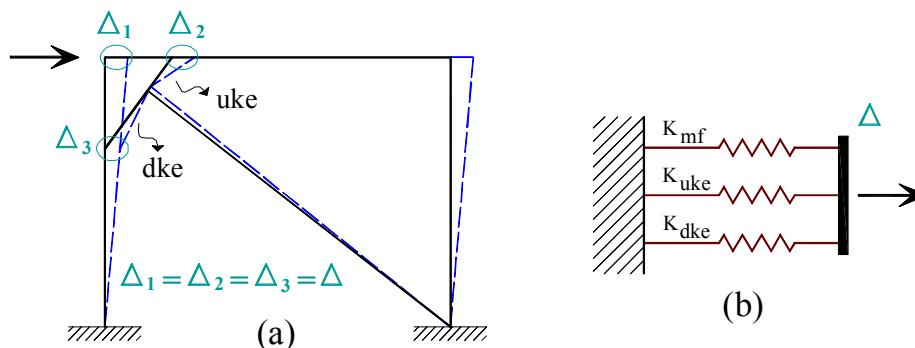
شکل ۱۰: سختی غیر الاستیک قاب KBF (پس از تسلیم مصالح، در ناحیه سخت شدگی کرنش) (a) قاب مهار بندی شده زانویی (b) مدل سختی غیر الاستیک قاب
