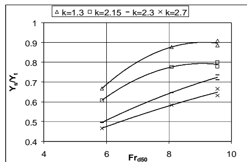
شکل ۳: تغییر حداکثر عمق حفرة آبستنگی با تغییرات عدد فرود مصالح Fr_{d50}
