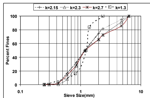
شکل ۲: منحنی دانه بندی مصالح مورد استفاده در آزمایش ها.
