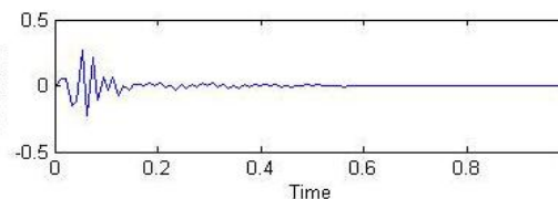
شکل ۹: تاریخچه شتاب - زمان در فاصله ۳/۵ متری از تکیه گاه چپ در تمامی نمونه‌ها.
