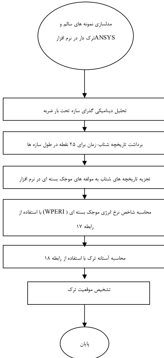
شکل ۳: فلوجارت نشان دهنده پروسه عملیات شناسایی ترک.
