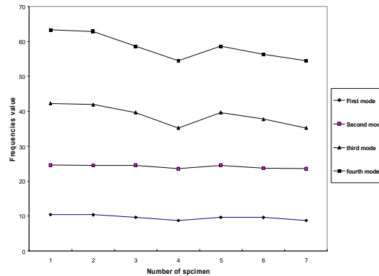
شکل ۷: تغییرات فرکانسی نمونه‌ها در چهار فرکانس اول.
