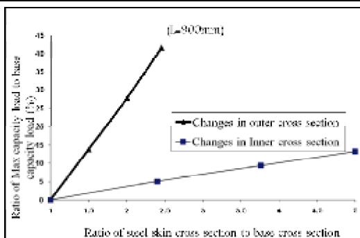
شکل ۲۴: میزان افزایش ظرفیت باربری ظرفیت باربری نمونه های کوتاه به ازای افزایش در سطح مقطع جداره‌ها.
