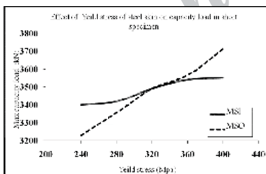
شکل ۱۰: اثر تنش تسلیم جداره‌ها بر روی حداکثر ظرفیت باربری در نمونه‌های کوتاه (ارتفاع ۷۵۰ mm).
