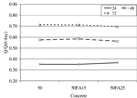
شکل 5: حرارت‌زایی بتن رده 50 حاوی خاکستر بادی.
