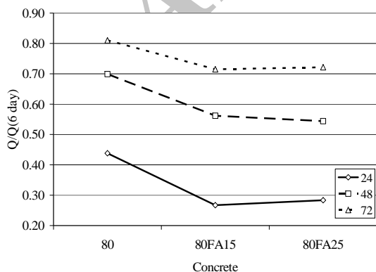
شکل 6: حرارت‌زایی بتن رده 80 حاوی خاکستر بادی.
