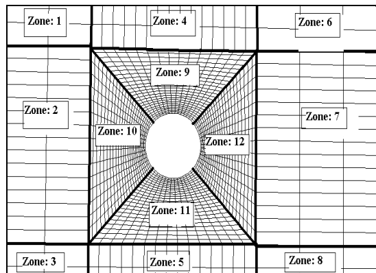
شکل ۱: تقسیم بندی مناطق حول پایه جهت تولید شبکه حل عددی نتایج
