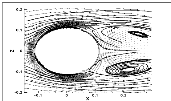
شکل ۴: نتایج شبیه سازی عددی: گردابه‌های ایجاد شده در ناحیه پشت پایه پل (نمای افقی)
