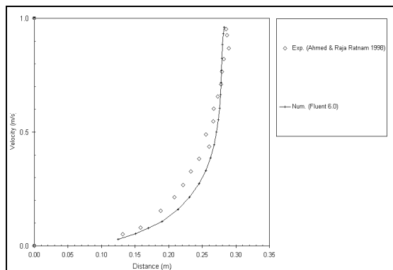
شکل ۹: مقایسه نتایج عددی با نتایج آزمایش احمد [۱۱] در فاصله ۳ برابر شعاع پایه در بالادست آن
