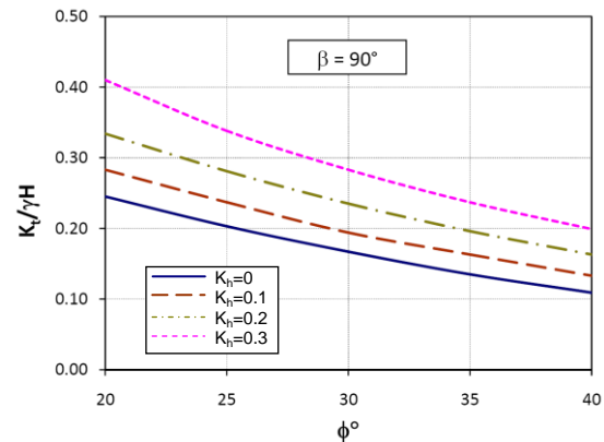
شکل 11: نیروی مورد نیاز جوشن نسبت به زاویه اصطکاک داخلی خاک و ضریب شتاب زلزله برای شیب 90 درجه
