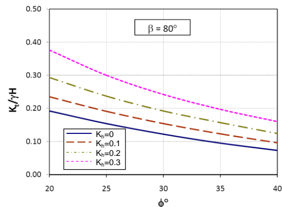
شکل 12: نیروی مورد نیاز جوشن نسبت به زاویه اصطکاک داخلی خاک و ضریب شتاب زلزله برای شیب 80 درجه
