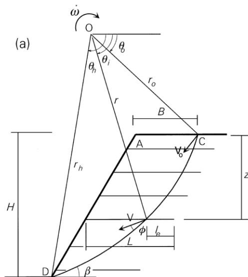
شکل 3: مکانیزم چرخشی اسپیرال لگاریتمی [5]
