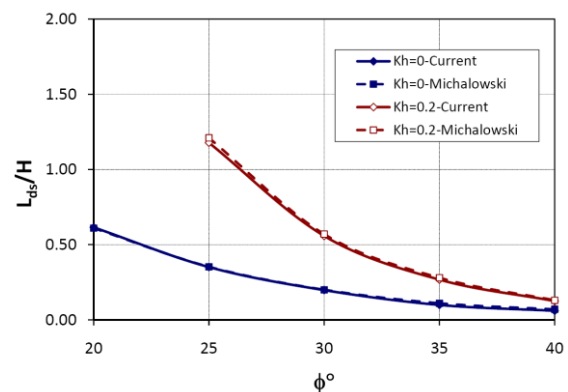
شکل 10: مقایسه طول جوشن‌های به دست آمده از الگوریتم حاضر با نتایج میخالفسکی در دو حالت استاتیکی و شبه استاتیکی برای شیروانی‌های قائم (مکانیزم لغزش مستقیم)
