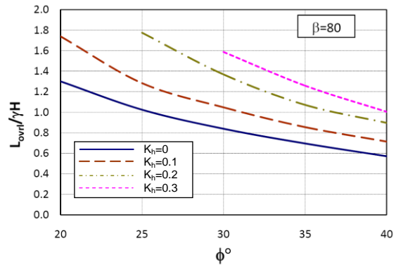
شکل 16: طول مورد نیاز جوشن برای مقابله با گسیختگی کلی نسبت به زاویه اصطکاک داخلی خاک و ضریب شتاب زلزله برای شیب 80 درجه
