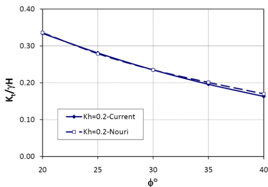
شکل 8: مقایسه نیروی جوشن بدست آمده از الگوریتم حاضر با نتایج نوری و همکاران در حالت شبه استاتیکی برای شیب قائم ( k_h = 0.2 )
