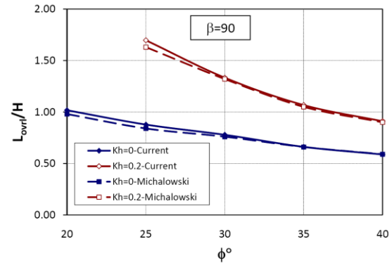
شکل 9: مقایسه طول جوشن‌های بدست آمده از الگوریتم حاضر با نتایج میخالفسکی در دو حالت استاتیکی و شبه استاتیکی برای شیروانی‌های قائم (مکانیزم گسیختگی کلی)
