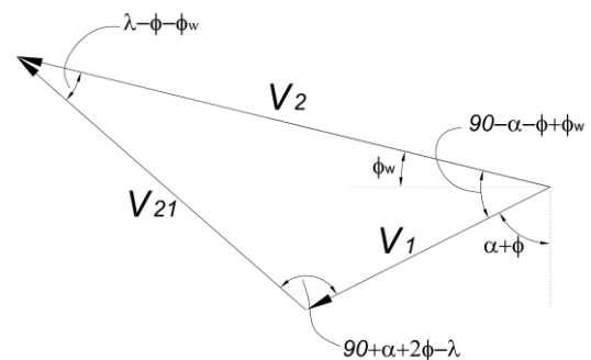
شکل 6: هداگراف سرعت برای مکانیزم لغزش مستقیم
