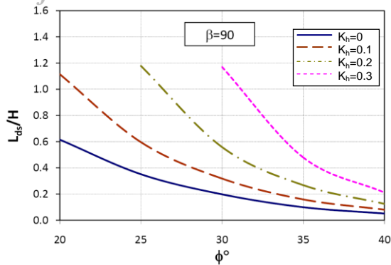
شکل 13: طول مورد نیاز جوشن برای مقابله با لغزش مستقیم نسبت به زاویه اصطکاک داخلی خاک و ضریب شتاب زلزله برای شیب 90 درجه
