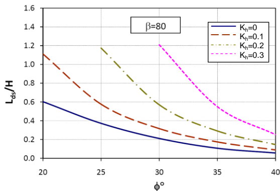
شکل 14: طول مورد نیاز جوشن برای مقابله با لغزش مستقیم نسبت به زاویه اصطکاک داخلی خاک و ضریب شتاب زلزله برای شیب 80 درجه
