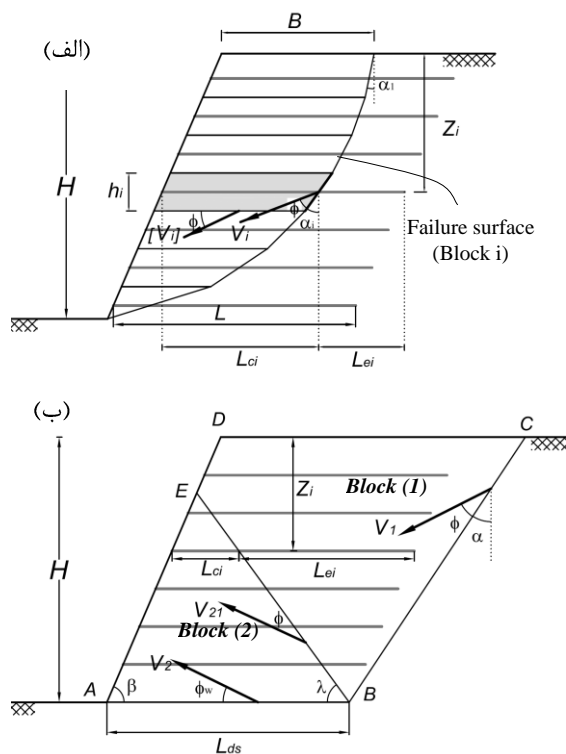
شکل 4: مکانیزم‌های گسیختگی مورد استفاده در تحقیق حاضر
