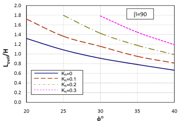
شکل 15: طول مورد نیاز جوشن برای مقابله با گسیختگی کلی نسبت به زاویه اصطکاک داخلی خاک و ضریب شتاب زلزله برای شیب 90 درجه
