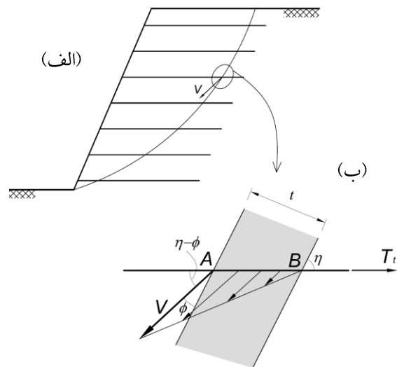
شکل 1: بردار سرعت در محل قطع جوشن با سطح گسیختگی [8]
