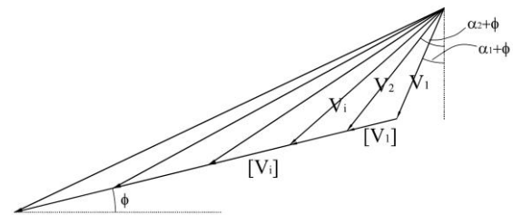
شکل 5: هدرگراف سرعت برای مکانیزم چند بلوکی مورد استفاده
