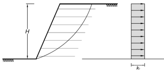
شکل 2: شیروانی با توزیع یکنواخت جوشن‌ها در ارتفاع
