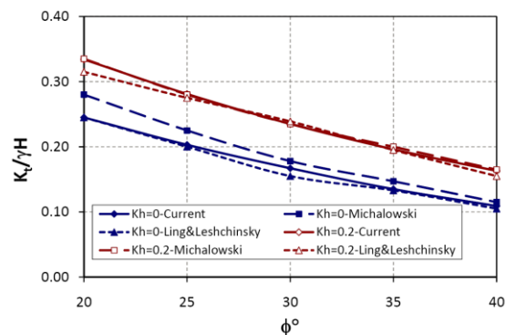
شکل 7: مقایسه نیروی جوشن بدست آمده از الگوریتم حاضر با نتایج میخالفسکی و لینگ در دو حالت استاتیکی و شبه استاتیکی برای شیب قائم
