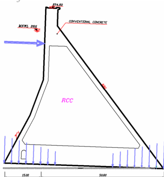
شکل 12: تأثیر بلند شدگی قاعده سد بر روی تنش‌های فشاری
