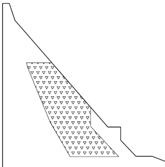
شکل 2: در محدوده هاشور زده از مقطع سد Miel I ملات بستر استفاده نشد [10]
