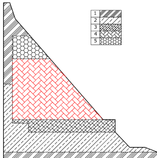
شکل 1: مقطع سد Miel I و نحوه ناحیه‌بندی طرح اختلاط و ملات بستر [3]
