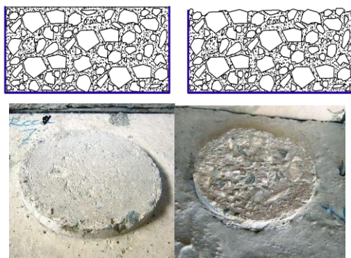
شکل 3: سطح درزه قبل و بعد از مضرس کرد
