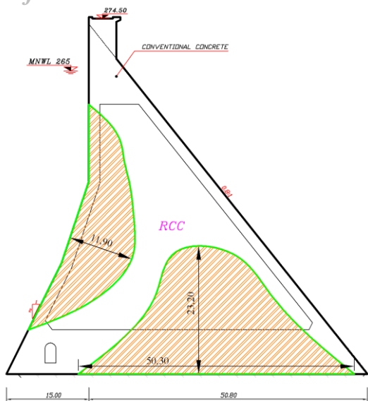
شکل 9: محدوده هاشور خورده، در حالت C=0.42 MPa از لحاظ برشی نیاز به بهسازی درزه ندارد.
