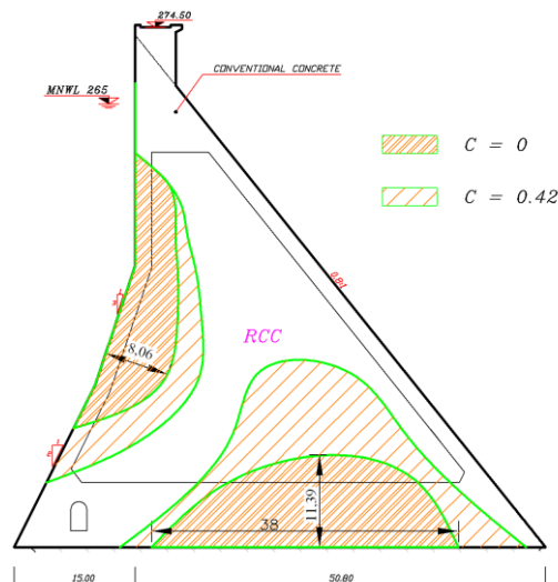
شکل 11: تأثیر مقدار چسبندگی ناحیه‌ای از مقطع سد از لحاظ برشی نیاز به به‌سازی درزه ندارد
