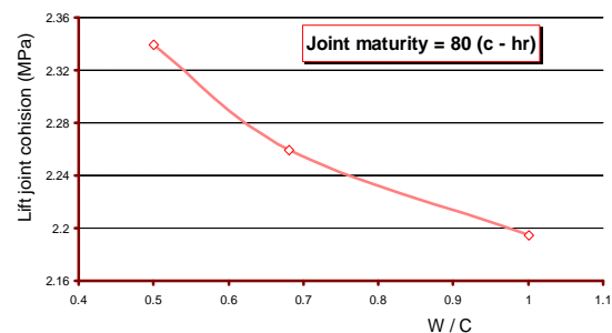
شکل 4: تأثیر دوغاب‌ها با نسبت آب به سیمان مختلف روی مقاومت چسبندگی
