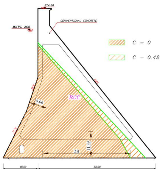
شکل 13: تخمین ناحیه‌ای از مقطع سد از لحاظ برشی نیاز به به‌سازی درزه ندارد، با در نظر گرفتن بلندشدگی قاعده سد از پی
