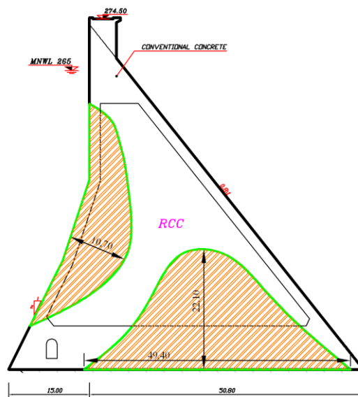
شکل 7: محدوده هاشور خورده، در حالت C=0.33 MPa از لحاظ برشی نیاز به بهسازی درزه ندارد.
