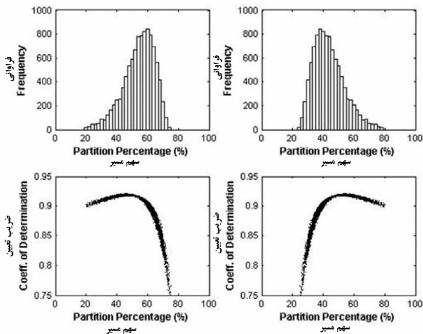
نمودار ۱۳- الف: فراوانی درصد حجم عبوری جریان از مسیر تند ب: فراوانی درصد حجم عبوری جریان از مسیر کند ج: حجم عبوری از مخزن مسیر تند و ضریب تعیین مدل د: حجم عبوری از مخزن مسیر کند و ضریب تعیین مدل
