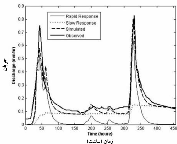
نمودار ۱۱- هیدروگراف‌های شبیه‌سازی شده، مشاهداتی و مسیرهای جریان تند و کند
