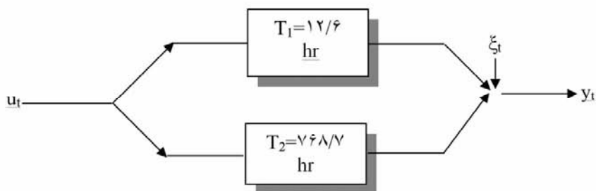
نمودار ۱۰- روندیابی بارش مؤثر از طریق مسیرهای موازی
