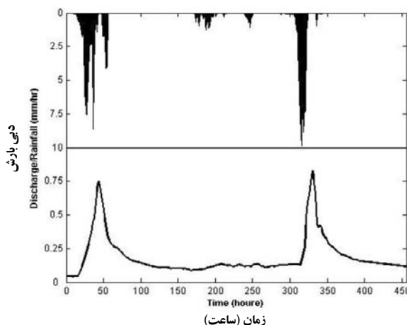
نمودار ۱- سری‌های زمانی بارش - رواناب - حوضه کارون علیا، ۲۶ اسفند ۱۳۷۶ الی ۱۵ فروردین ۱۳۷۷
