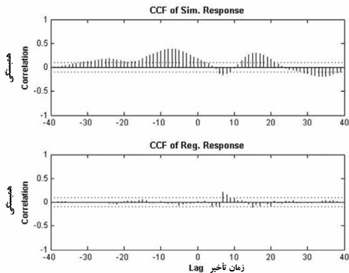
نمودار ۹- همبستگی در عرض مانده‌ها ب: پاسخ رگرسیون الف: پاسخ شبیه‌سازی
