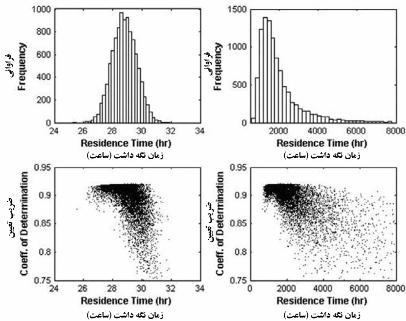
نمودار ۱۲- الف: فراوانی زمان نگاهداشت مخزن مسیر کند ب: فراوانی زمان نگاهداشت مخزن مسیر تند ج: زمان نگاهداشت مخزن مسیر کند و ضریب تعیین د: زمان نگاهداشت مخزن مسیر تند و ضریب تعیین
