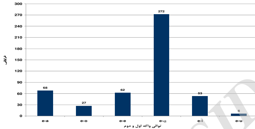
شکل ۳ فراوانی توالی v_2 -e در واژه‌هایی با ساختار هجایی (C) V_1.CV_2C
