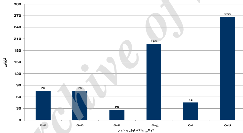
شکل ۴ فراوانی توالی v_2 -o در واژه‌هایی با ساختار هجایی (C) V_1.CV_2C
