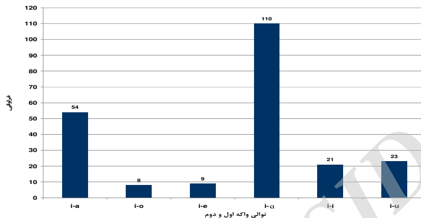
شکل ۶ فراوانی توالی i - v 2 در واژه‌هایی با ساختار هجایی (C) CV 1 .CV 2 C
