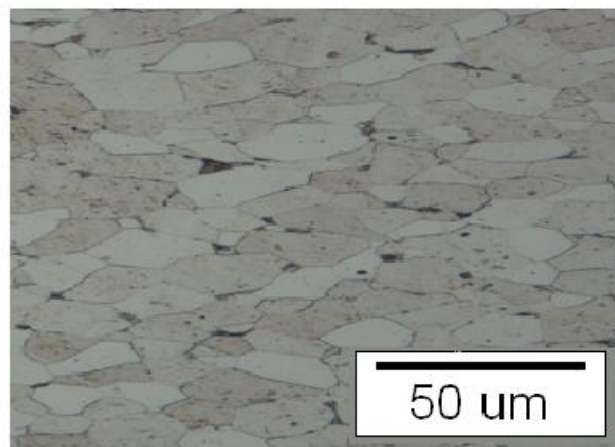
شکل ۲: ریزساختار ورق St14
