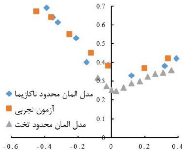
شکل ۱۶: نمودار حد شکل‌دهی مدل تخت، ناکازیمبا و تجربی
