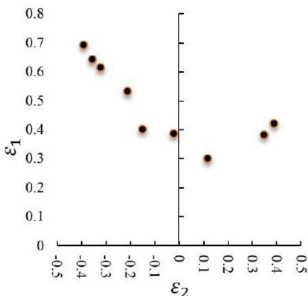
شکل ۱۲: نمودار حد شکل‌دهی مدل المان محدود ناکازیم
