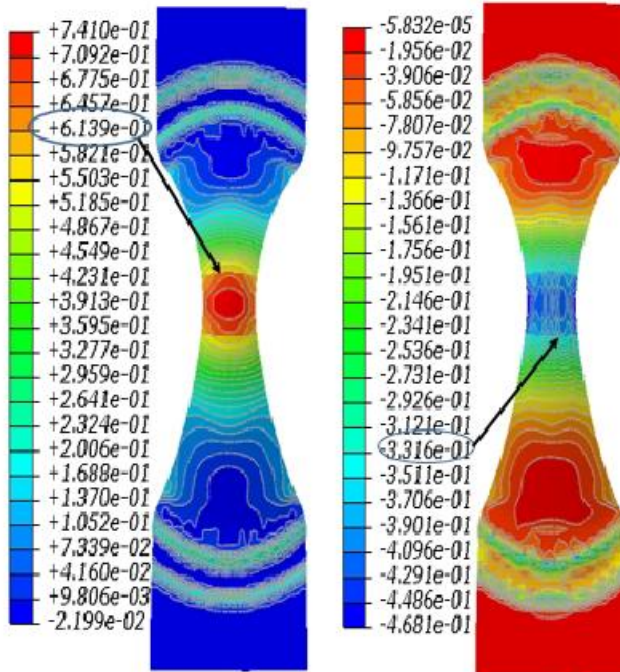
شکل ۹: کانتور کرنش در شرایط گالیبره شده مد کشش
