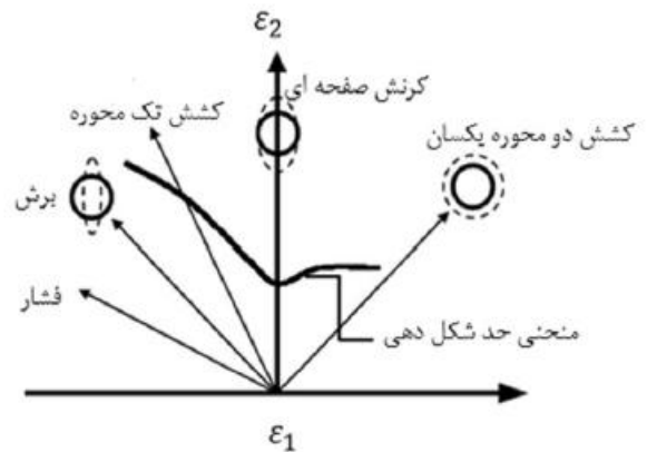
شکل ۱: شماتیکی از نمودار حد شکل‌دهی
