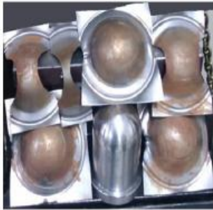
شکل ۶: شش نمونه نمونه‌های آزمون ناگازیمما و نمونه‌ها بعد از تغییر شکل
