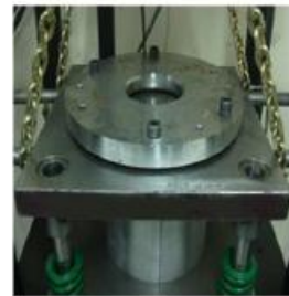
شکل ۵: قالب آزمون ناگازیمما
