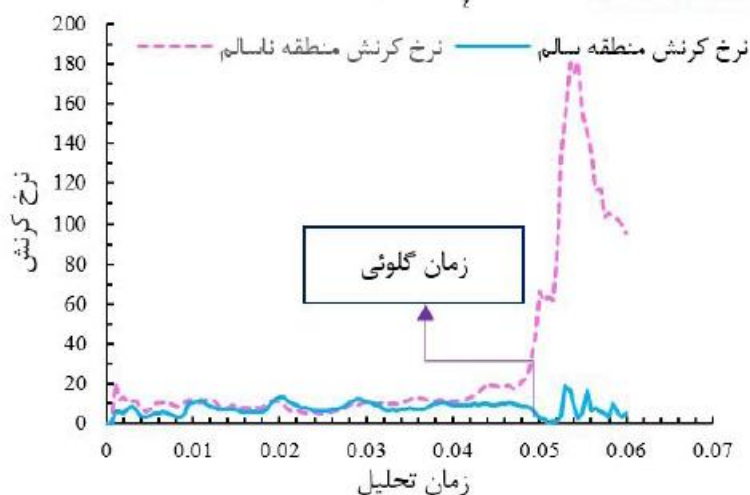
شکل ۱۵: کانتور کرنش و نحوه تعیین زمان گلوئی موضعی برای مد کرنش صفحه‌ای
