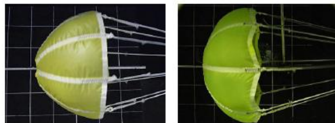
الف- کانوی نفوذپذیر ب- کانوی نفوذناپذیر
