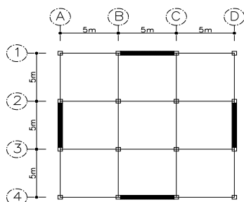
شکل (۱): پلان طبقات سازه های مدل شده
