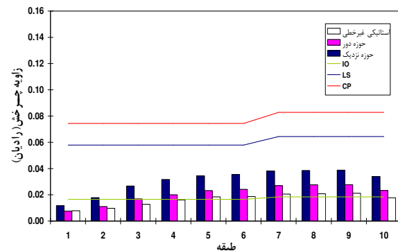
نمودار (۱): بررسی عملکرد تیرهای سازه ۱۰ طبقه
