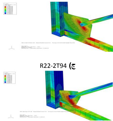
شکل (۸): حالت نهایی نمونه‌ها
