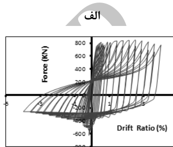
شکل (۶): نمودار هیستریزیس و تغییر شکل نهایی حاصل از تحلیل نمونه R22-2T94
