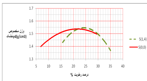
شکل (۳): اثر توام حداکثر مقدار الیاف و آهک مصرفی بر مشخصات تراکمی خاک
