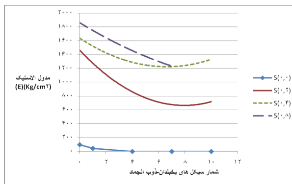
شکل (۱۱): نمودار تغییرات مدول الاستیک در مقابل دوره‌های انجماد و ذوب برای تیمارهای تثبیت شده با آهک
