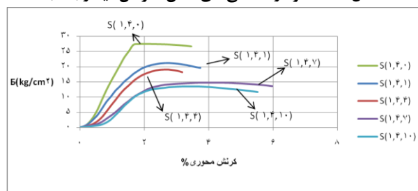
شکل (۲۱): نمودار منحنی‌های تنش-کرنش تیمار S(1,4)
