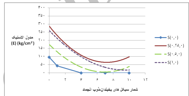
شکل (۱۵): نمودار تغییرات مدول الاستیک در مقابل دوره‌های انجماد-ذوب یخبندان برای تیمارهای تسلیح شده با الیاف پلی پروپیلن
