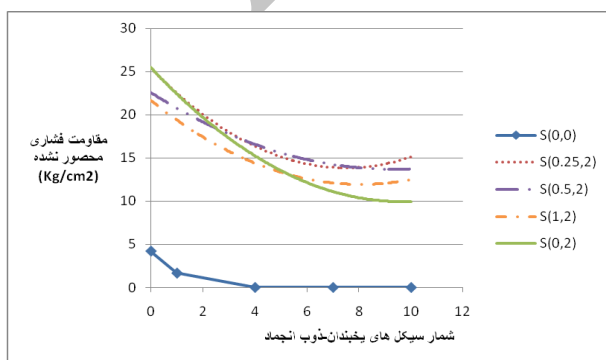
شکل (۵): نمودار تغییرات مقاومت فشاری محصور نشده در مقابل دوره‌های انجماد - ذوب یخبدان برای نمونه‌های تثبیت
