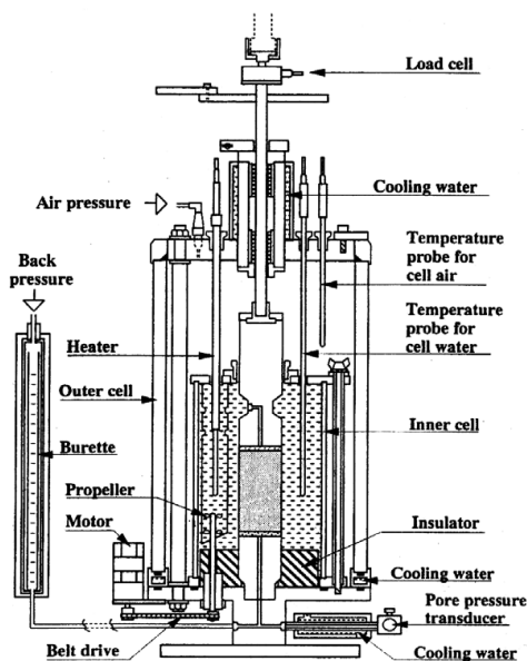
شکل (۳): دستگاه سه محوری با کنترل دما ساخت کانتی واتاناکول و همکاران
