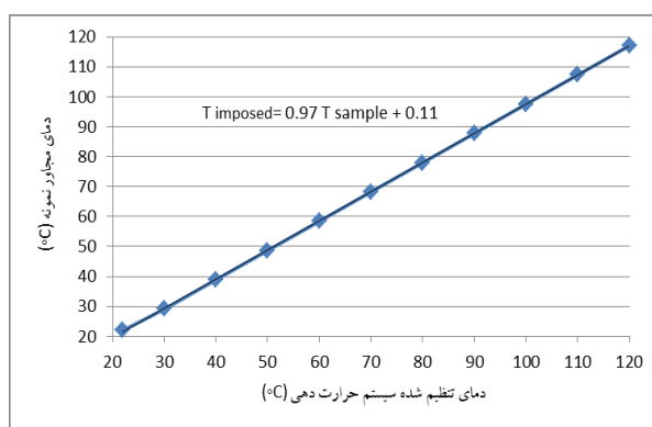
شکل (۶): رابطه دمای تنظیم شده در سیستم حرارت دهی و دمای قرائت شده مجاور نمونه
