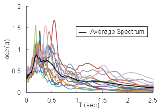
شکل (۵): طیف‌های پاسخ شتاب حاصل از تحلیل غیرخطی
