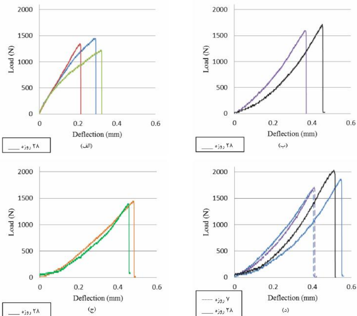
شکل ۱: منحنی‌های بار - جابجایی آزمایش خمش سه نقطه‌ای: الف) نمونه‌های CM1 (الف) نمونه‌های CM2 (ب) نمونه‌های CM3 (ج) نمونه‌های CM4 (د) نمونه‌های CM4
