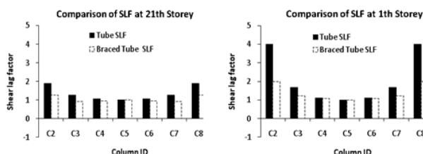
شکل ۱۶: نرخ تغییرات ضریب تاخیر برشی در ستون‌های بال کششی سازه در طبقات ۲۱، ۱ و ۶۱ (الف تا ج) و نرخ تغییرات ضریب تاخیر برشی در طبقات مختلف بال کششی (د) سیستم لوله مه‌ار بندی شده (ابر-مه‌ار بند)
