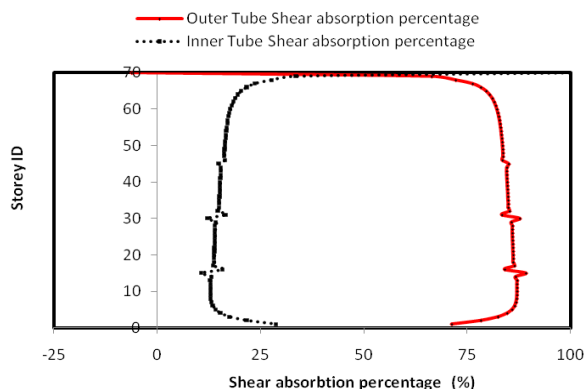
شکل ۸: درصد جذب برش لوله خارجی و لوله داخلی از کل نیروی برش طبقه
