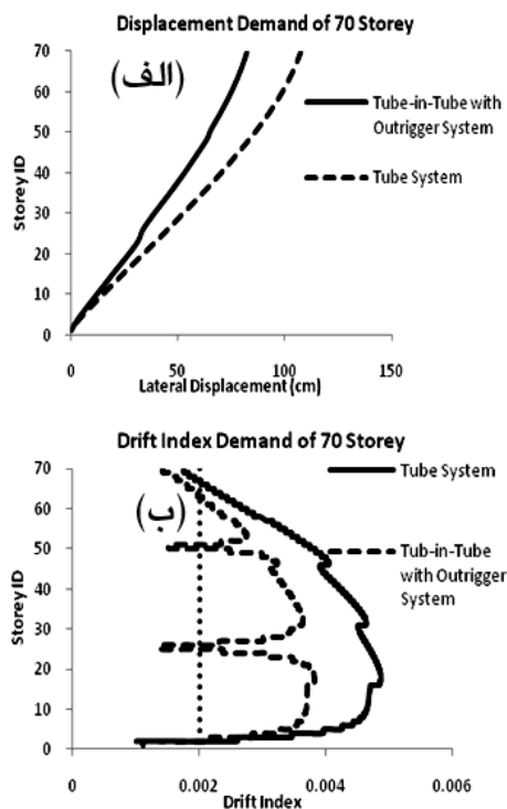
شکل ۱۲: مقایسه الف) تغییر مکان مطلق طبقات ب) اندیس رانش بین طبقه‌ای در دو سازه لوله تنها و لوله در لوله با کلاhek خرابایی
