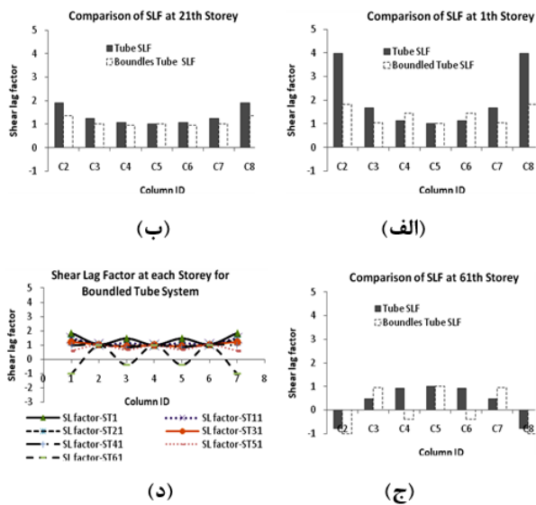
شکل ۱۹: تغییرات ضریب تاخیر برشی در ستون‌های بال کششی سازه در طبقات ۲۱، ۱ و ۶۱ (الف تا ج) و تغییرات ضریب تاخیر برشی در طبقات مختلف بال کششی (د) سیستم لوله در لوله دسته بندی شده
