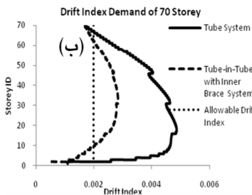
شکل ۹: مقایسه الف) تغییر مکان مطلق طبقات (ب) اندیس رانش بین طبقه‌ای در دو سازه لوله تنها و لوله در لوله با هسته داخلی
