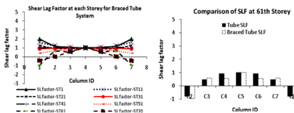
شکل ۱۶: نرخ تغییرات ضریب تاخیر برشی در ستون‌های بال کششی سازه در طبقات ۲۱، ۱ و ۶۱ (الف تا ج) و نرخ تغییرات ضریب تاخیر برشی در طبقات مختلف بال کششی (د) سیستم لوله مه‌ار بندی شده (ابر-مه‌ار بند)
