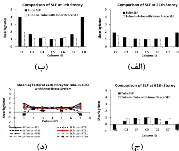
شکل ۱۰: نرخ تغییرات ضریب تاخیر برشی در ستون‌های مستقر در بال کششی سازه در طبقات ۱، ۲۱ و ۶۱ (شکل‌های الف تا ج) و نرخ تغییرات ضریب تاخیر برشی در طبقات مختلف بال کششی (شکل د) سیستم لوله در لوله با هسته داخلی
