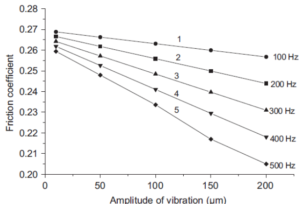
شکل ۵: تغییرات ضریب اصطکاک با تغییرات دامنه ارتعاش در فرکانس های مختلف \omega = 1/17 \text{ m/s} ، سرعت ارتعاش، 10 \text{ N} نیروی نرمال، 0.2 \mu\text{m} زبری تماس و 50\% رطوبت نسبی نمونه آزمایش: الیاف شیشه [۱۴]
