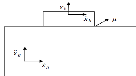
شکل ۸: مدل تحلیل شده جسم صلب بر روی پی لغزشی
