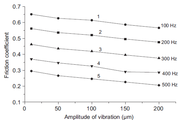
شکل ۶: تغییرات ضریب اصطکاک با تغییرات دامنه ارتعاش در فرکانس های مختلف \omega = 1/17 \text{ m/s} ، سرعت ارتعاش، 10 \text{ N} نیروی نرمال، 0.2 \mu\text{m} زبری تماس و 50\% رطوبت نسبی نمونه آزمایش: فولاد نرم [۱۴]
