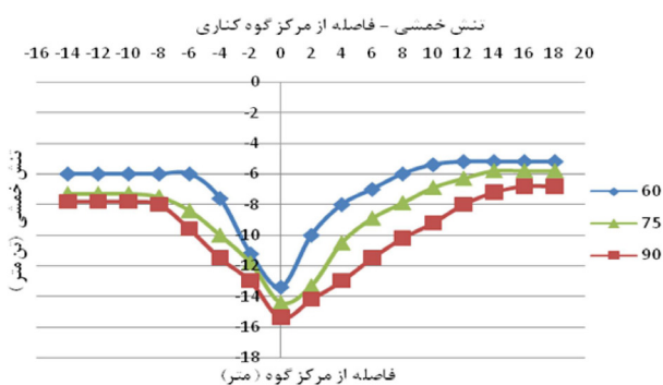
شکل ۱۴: تنش خمشی دیواره-فاصله از مرکز گوه برای مقادیر مختلف زاویه تقاطع
