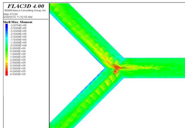
شکل ۱۰: کانتور ممان روی لاینینگ تاج تونل-تقاطع ۹۰ درجه
