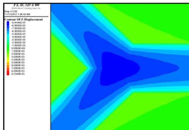
شکل ۶: کانتور جابجایی تاج در تراز ۳۵۷ متر زیر سطح زمین - تقاطع ۹۰ درجه
