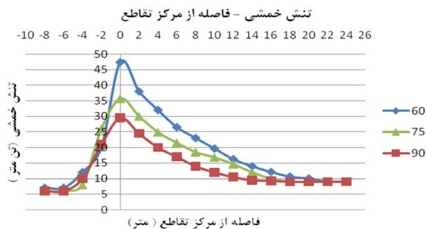
شکل ۱۲: نمودار تنش خمشی روی تاج-فاصله از مرکز تقاطع برای مقادیر مختلف زاویه تقاطع
