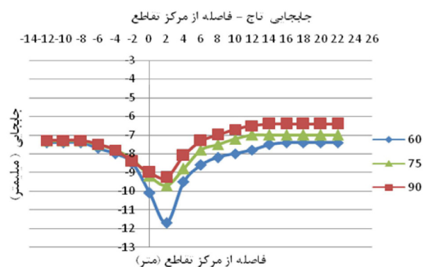
شکل ۱۱: نمودار جابه‌جایی تاج-فاصله از مرکز تقاطع برای مقادیر مختلف زاویه تقاطع
