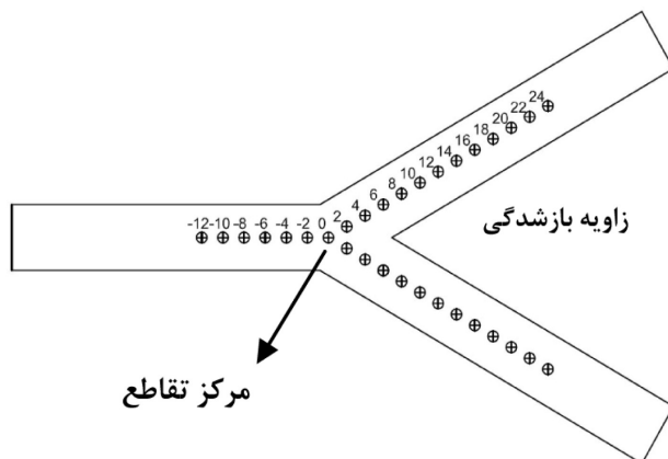
شکل ۴: نمایش محل نقاط بحرانی در تاج تونل
