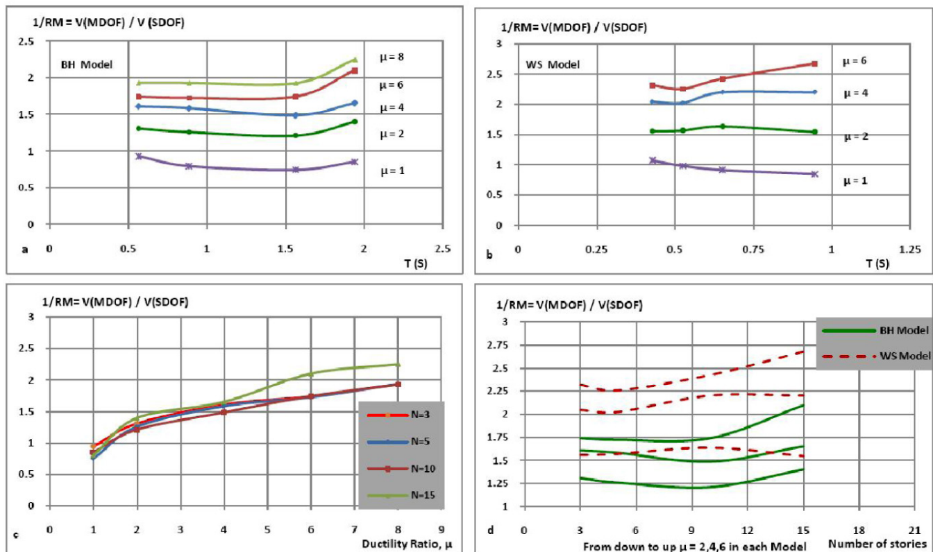
شکل ۲: a,b,d) طیف‌های ضریب اصلاحی برآورد شده بر حسب زمان تناوب سازه ( T ) و تعداد طبقات ( N ) در دو سازوکار BH و WS؛ c) روند تغییرات ضریب اصلاحی بر حسب نسبت شکل‌پذیری در سازه‌های مختلف
