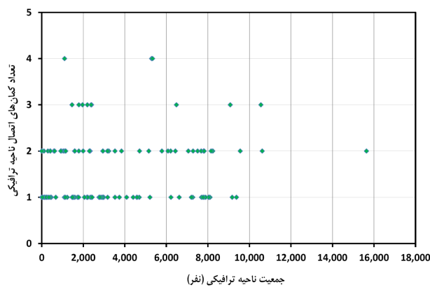
شکل ۴: پراکنش تعداد کمان‌های اتصال با جمعیت ساکن ناحیه Fig. 4. Dispersion of the Number of Connectors vs. TAZ Population
