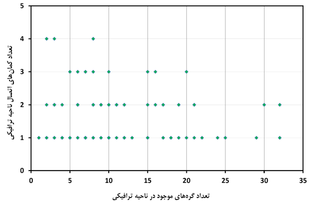
شکل ۷: پراکنش تعداد کمان‌های اتصال با تعداد گره‌های ناحیه
