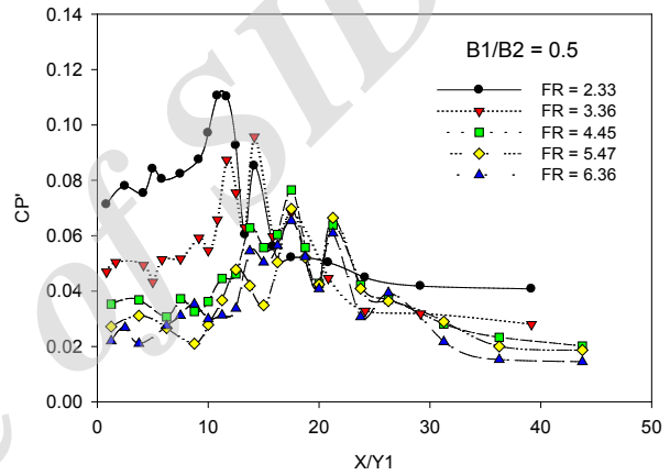
شکل ۷: (ب) تغییرات ضریب C'p در نسبت واگرایی ۰/۵ Fig.7. (b) Variation of C'p for \beta=0.5
