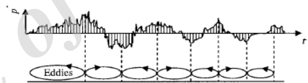
شکل ۱-الف: گرداب‌ها در مقیاس بزرگ و فرکانس کم
