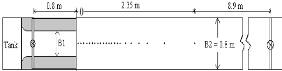
شکل ۴: پلان کانال آزمایشگاه
