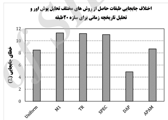
شکل ۲۱: خطای ناشی از روش‌های مختلف تحلیل استاتیکی غیرخطی در محاسبه جابجایی طبقات سازه ۲۰ طبقه Fig. 21. 20 story model displacement error of NTHA in comparison with NSP method
