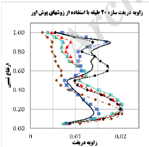
شکل ۱۲: نمودار زاویه دررفت طبقات سازه ۲۰ طبقه
