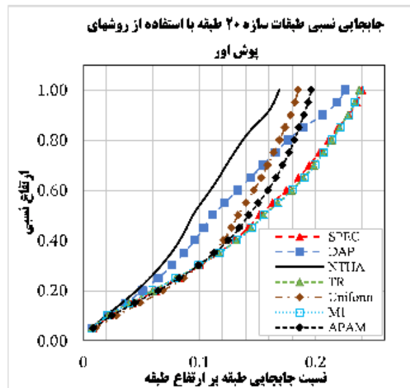
شکل ۱۱: نمودار جابجایی طبقات سازه ۲۰ طبقه
