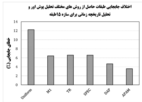
شکل ۱۹: خطای ناشی از روش‌های مختلف تحلیل استاتیکی غیرخطی در محاسبه جابجایی طبقات سازه ۱۵ طبقه Fig. 19. 15 story model displacement error of NTHA in comparison with NSP method
