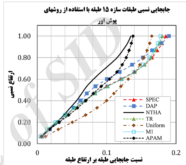
شکل ۹: نمودار جابجایی طبقات سازه ۱۵ طبقه
