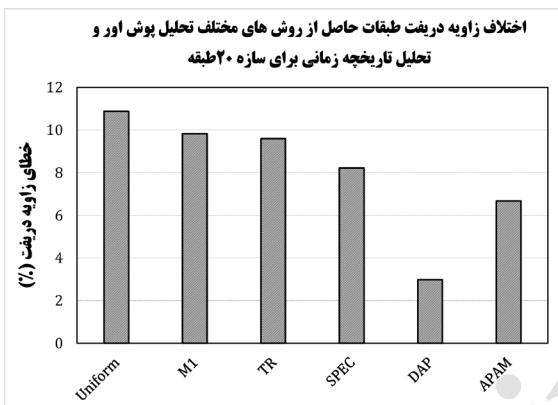
شکل ۲۲: خطای ناشی از روش‌های مختلف تحلیل استاتیکی غیرخطی در محاسبه زاویه دررفت طبقات سازه ۲۰ طبقه Fig. 22. 20 story model drift angle error of NTHA in comparison with NSP method
