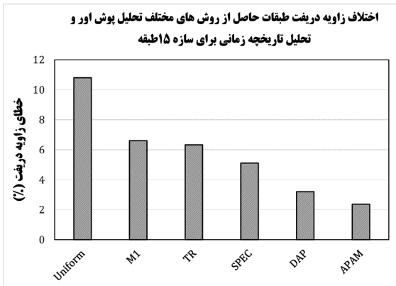
شکل ۲۰: خطای ناشی از روش‌های مختلف تحلیل استاتیکی غیرخطی در محاسبه زاویه دررفت طبقات سازه ۱۵ طبقه Fig. 20. 15 story model drift angle error of NTHA in comparison with NSP method
