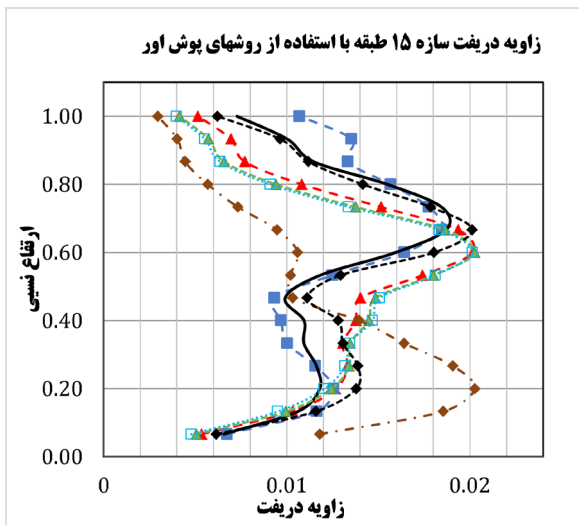
شکل ۱۰: نمودار زاویه دررفت طبقات سازه ۱۵ طبقه
