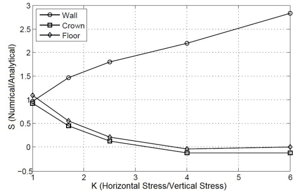
شکل ۱۷: نسبت حل عددی به تحلیلی در مقابل نسبت تنش‌های برجا، برای تونل عمیق (عمق ۳۰ متری)
