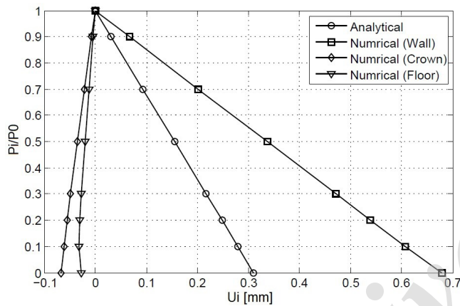
شکل ۹: منحنی‌های پاسخ زمین برای عمق ۲۲/۵ متری با K=4
