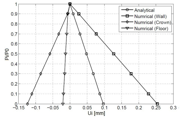
شکل ۶: منحنی‌های پاسخ زمین برای عمق ۵ متری با K=6
