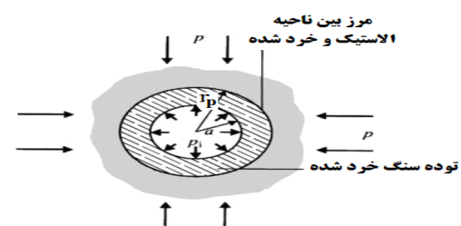
شکل ۱: مدل تحلیلی تحت تنش هیدرواستاتیک Fig. 1. The analytical model for the hydrostatic stress condition
