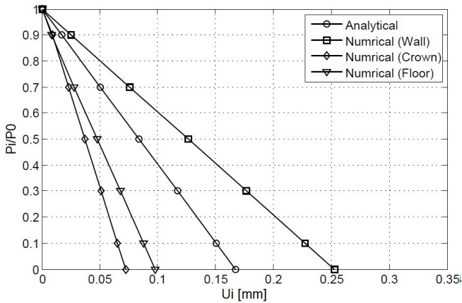
شکل ۸: منحنی‌های پاسخ زمین برای عمق ۲۲/۵ متری با K=1/7
