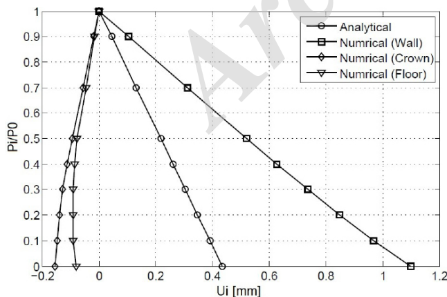
شکل ۱۰: منحنی‌های پاسخ زمین برای عمق ۲۲/۵ متری با K=6
