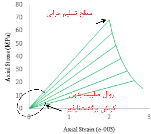
شکل ۴: منحنی تنش-کرنش شبیه سازی شده در آزمایش مقاومت فشاری تک محوره سنگ آهک اوولیتی با مدل رفتاری خرابی بدون لحاظ رفتار پلاستیک.
