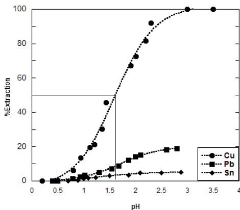
شکل ۱: درصد استخراج فلز مس، قلع و سرب برحسب pH از محلول اسید فلئوروبوریک در دمای ۲۵ °C توسط LIX984N ۲۰ درصد
