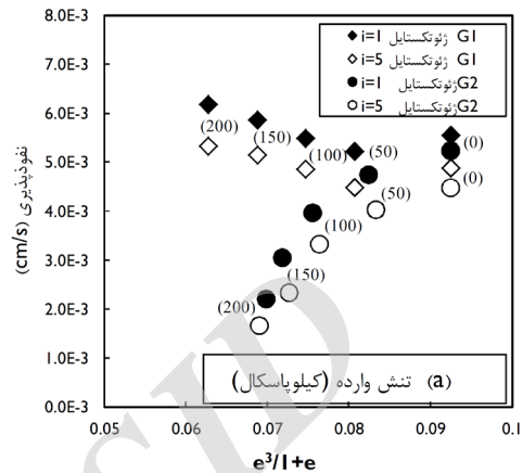
شکل ۱۵: تغییرات نفوذپذیری بر حسب e^3 / (1+e)
